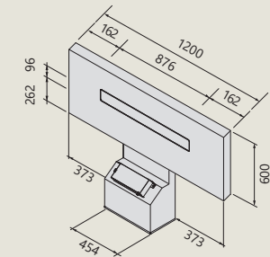
Διάσταση και θέση τρύπας εντοιχισμού
