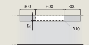
Διάσταση και θέση τρύπας εντοιχισμού
